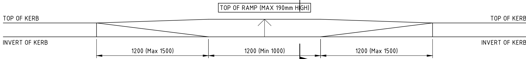
ELEVATION
